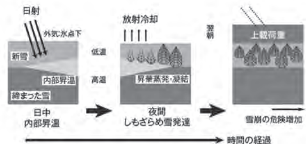
図14 しもぞらめ雪による弱層形成の模式図
