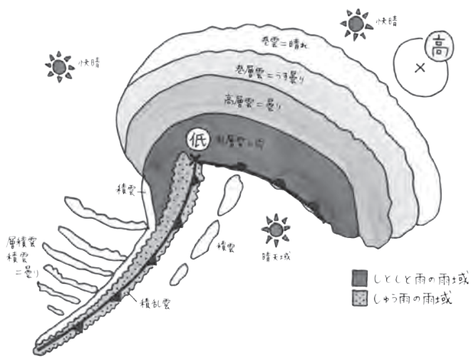
図6 低気圧と前線の位置
