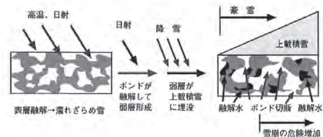
図18 濡れざらめ雪による弱層発生模式図
