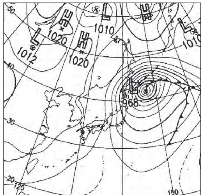
図9 白馬岳付近でガイドツアーの参加者4名が亡くなった日の天気図
