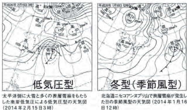
図1 低気圧型と冬型の天気図
