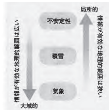
図21 雪崩ハザード評価の3つの要素
