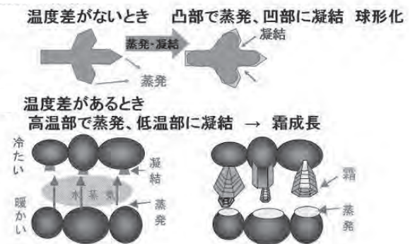
図5 積雪を不安定化する変化
