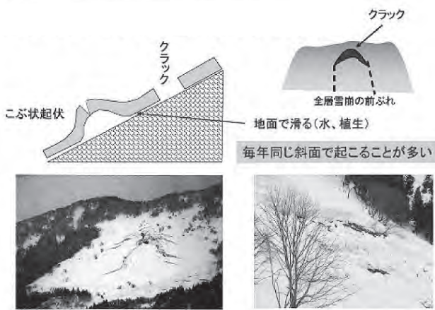
図19 全層雪崩の前兆現象
