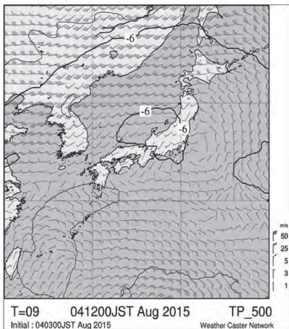
図15 中部山岳で落雷が多発した日の500hPa面の気温予想図
