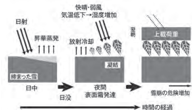
図15 表面霜による弱層形成の模式図
