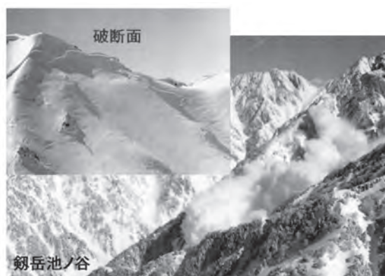
写真1 面発生表層雪崩と破断面(劔岳池ノ谷)
